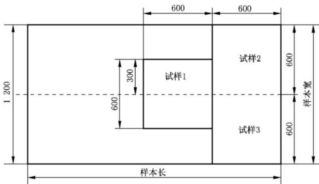
图 1 试样制作示意图
